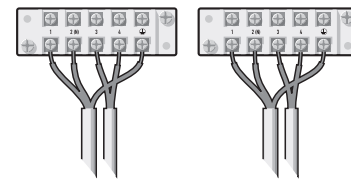
koncovka venkovního přístroje
